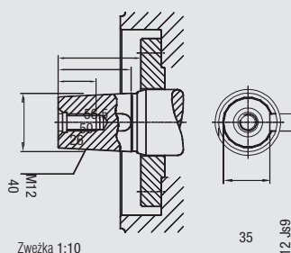
Rysunek wałka napędowego
